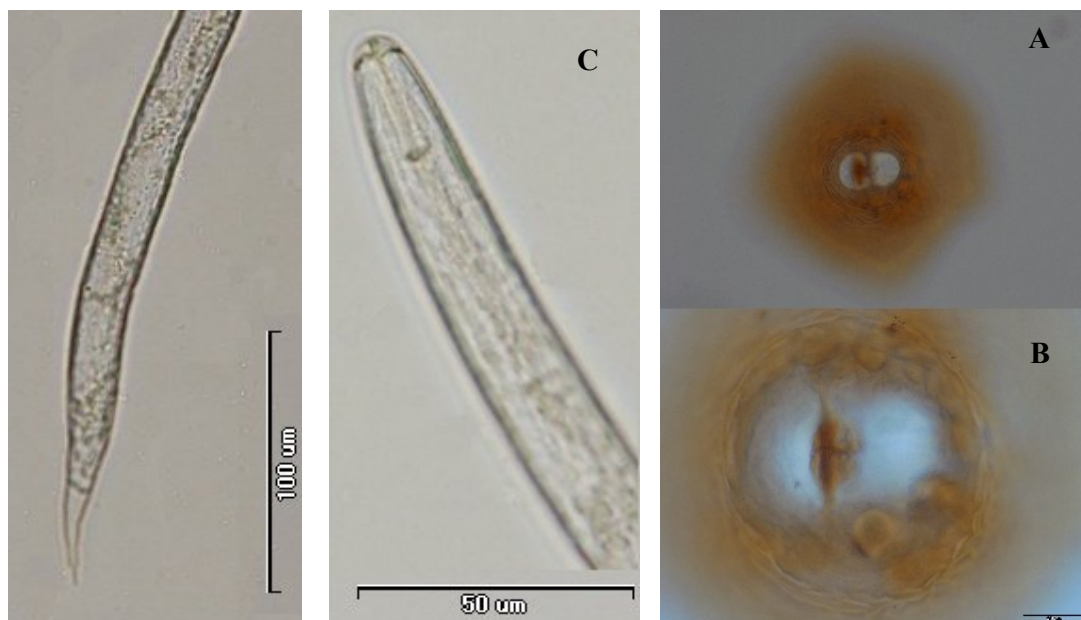
شکل ۱- (A) شکاف تناسلی، پنجره های خروجی لارو و باند های نگهدارنده واژن، (B) برآمدگی های کوتیکولی اطراف مخروط انتهایی سیست، (C) قسمت سر و استایلت، (D) شکل دم نماتد سیستی غلات گونه Heterodera filipjevi
